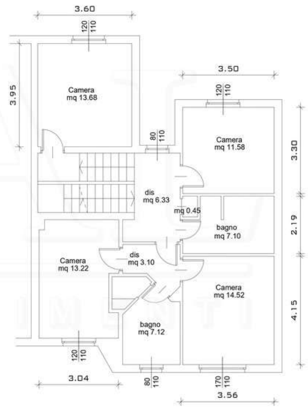
PIANO PRIMO
